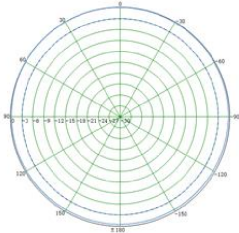
实测水平面方向图
