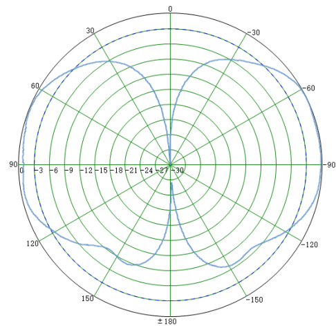
实测垂直面方向图
